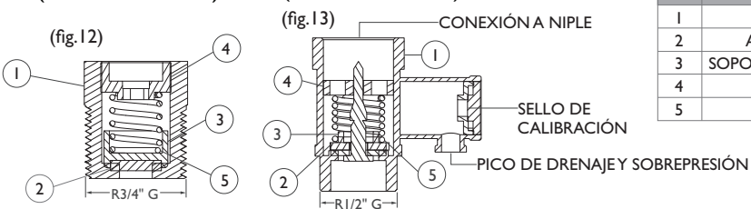
VÁLVULA DE ALIVIO (CONEXIÓN SUPERIOR)
