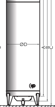
ELEC125 CS Para Colgar o Apoyar
