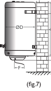
ELEC70 CS* 6 CI Para Colgar o Apoyar
